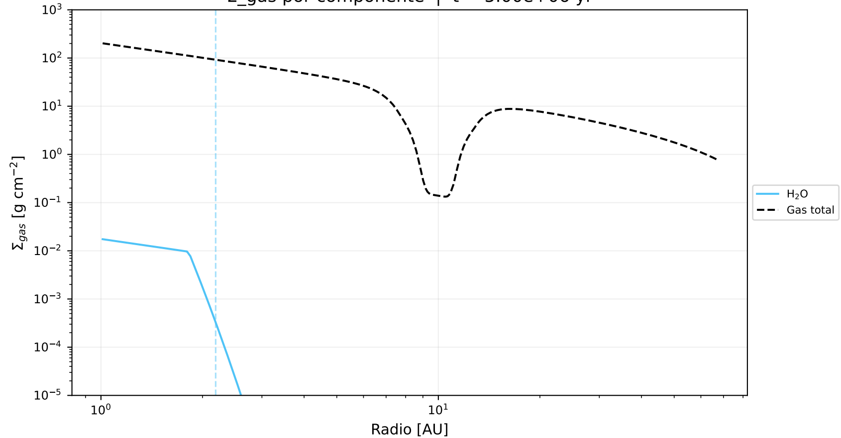
\Sigma_{\text{gas}} por componente | t = 5.00\text{e}+06 yr
